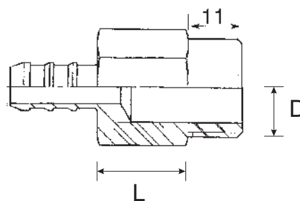
VMP - Maschio prolungato Virgilio - Ottone nichelato
